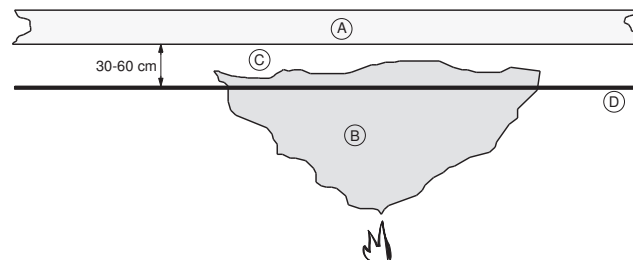
installatie_voor_rookpluim
