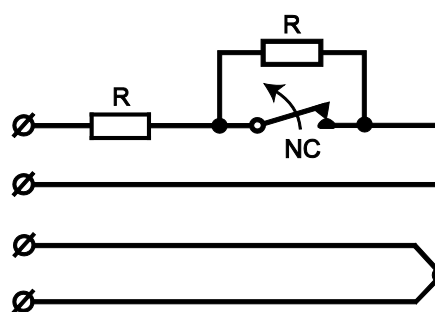
MC 240-S45-2R:
