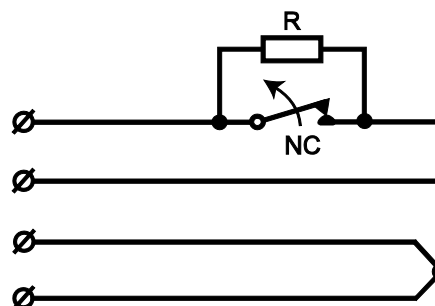
MC 240-S45-R:
