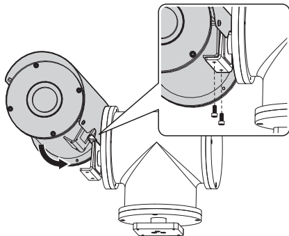
Abb. 7 S-N-Kopf Montage.
