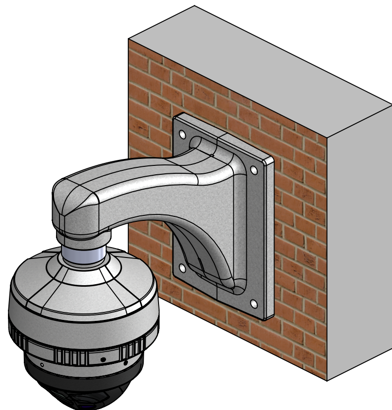
PENDANT MOUNT KIT - GEN-X SERIES PN (421-0069-00) SHEET 3/6
