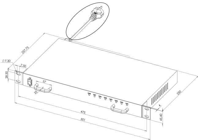
optional ADCAB3
